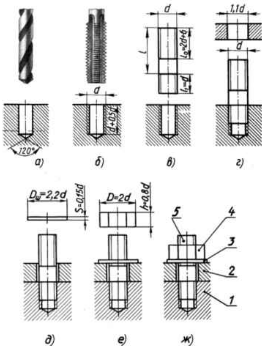
Расми 220. Тасвири содаи пайвасти санчоқӣ.
