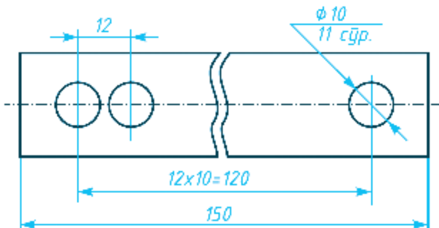
Расми 33. Нишон додани андозаҳои такроришаванда.
