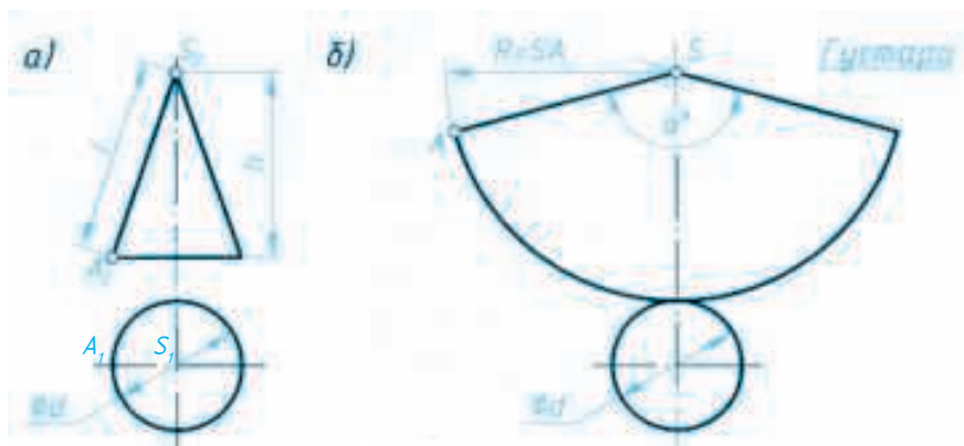
Расми 142. Сохтани нақшаи густараи сатҳи махрут: а-ду намуди махрут; б-густараи сатҳ.
