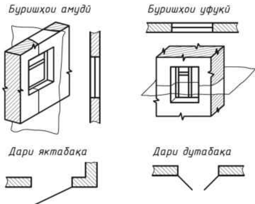
Расми 244. Ишоратҳои шартии ҷойҳои дару тиреза.
