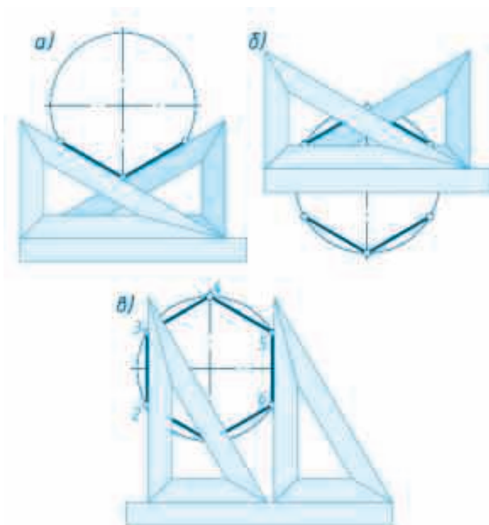
Расми 131. Тақсими давра ба шаш ҷиссаи баробар бо ёрии гунё ва хаткаш.
