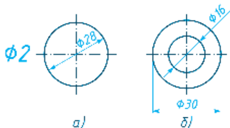
Расми 31. а -андозагузорӣ, б – андозагузори қутри давра.
