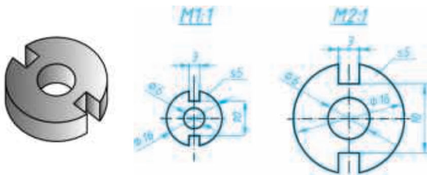
Расми 36. Нақшаи маснуот дар миқёсҳои гуногун.
