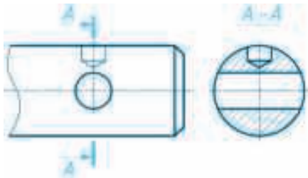
Расми 170. Бурише, ки дар он шакли сӯроҳ пурра нишон дода шудааст.
