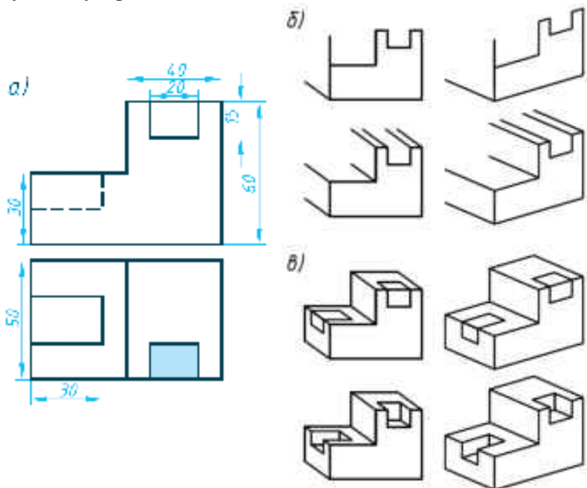
Расми 62. Сохтани проексияҳои аксонометрии ҷисмҳои ҳамворрӯя.
