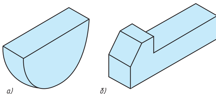
Рисми 225. Навъҳои гуваҳо: а - гуваи сегментӣ, б - гуваи фонашакл.
