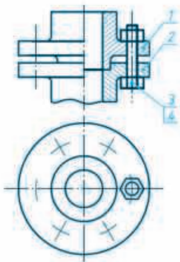
Расми 235. Тасвири шартҳои унсурҳои такроршаванда
