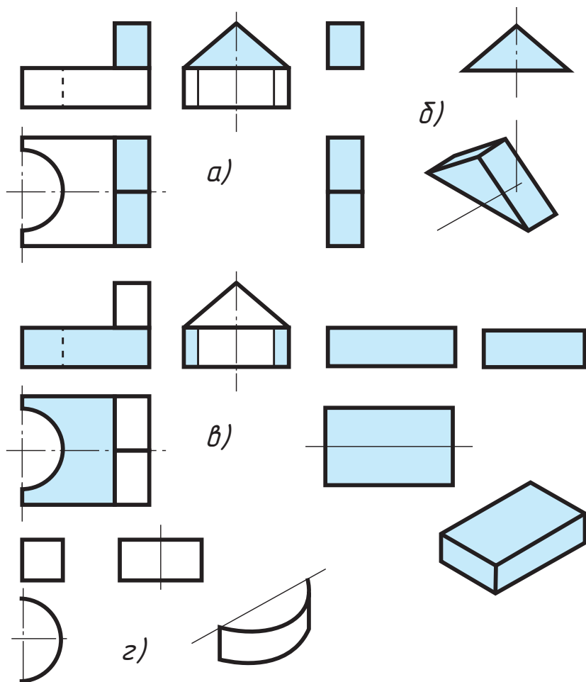
Рис. 105. Таҳлили шакли ҷисм.
