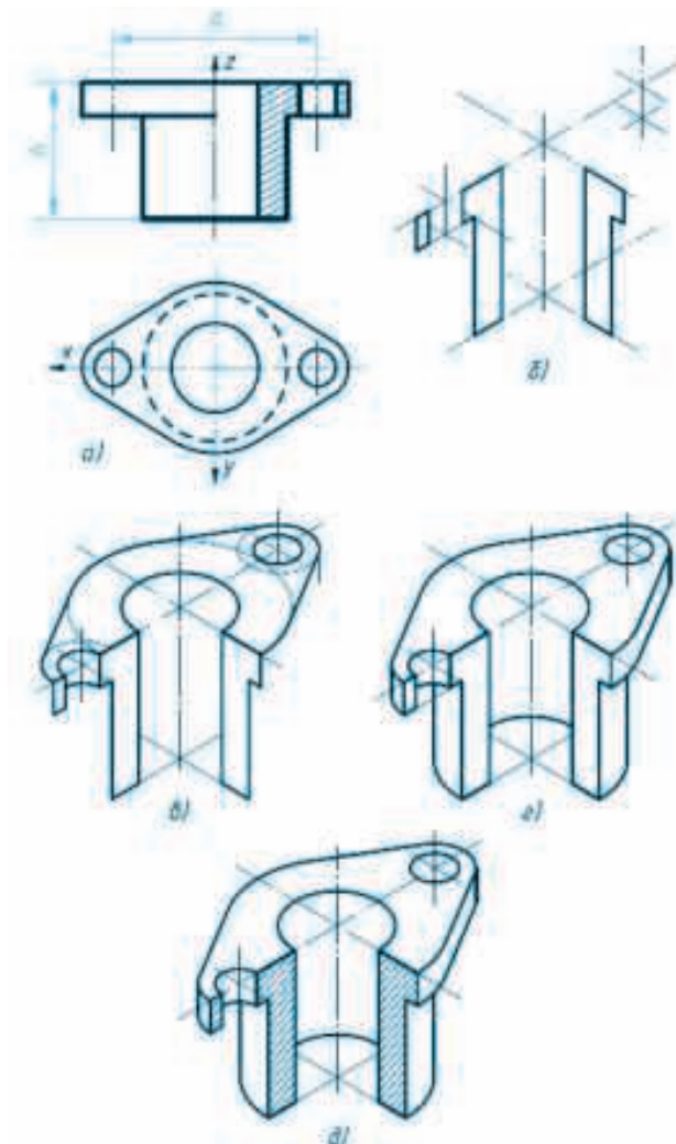
Расми 200. Пайдарпайии иҷрои буришгоҳ дар проексияи аксонометрӣ.
