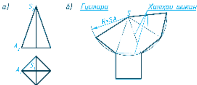
Расми 143. Сохтани нақшаи густараи сатҳи пирамида: а-ду намууди пирамида; б-густараи пирамида.
