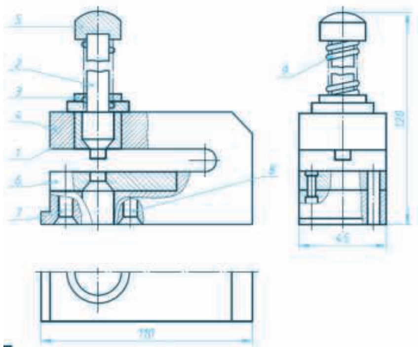
Расми 241. Нақшаи ҷиҳози сӯрохкунанда.
