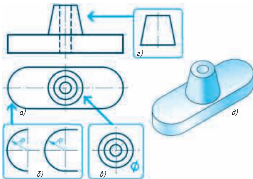
Расми 127. Таҳлили таркиби графикии тасвир.
