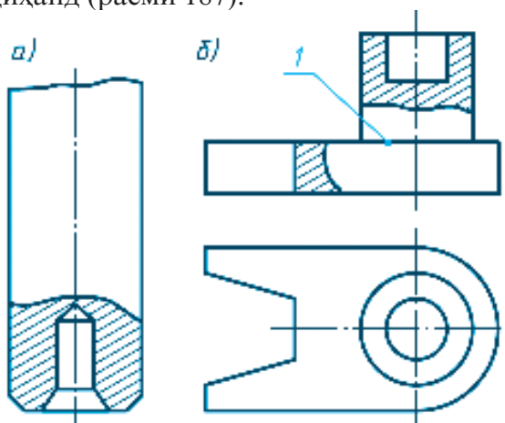
Расми 187. Тасвири буришгоҳи чузъӣ.
