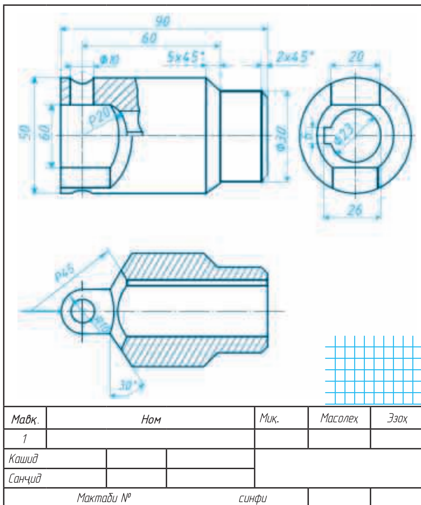
Расми 9. Ангора (эскиз).
