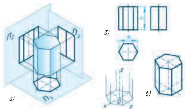
Расми 80: а-проексиясозӣ, б-нақшаи манишур дар системаи проексияҳои росткунҷа, в-проексияи изометрии манишур.
