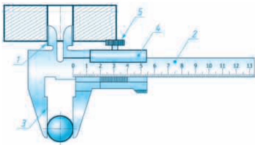
Расми 153. Чен кардани андозаҳо бо паргори хаткашдор (штангент-циркул).
