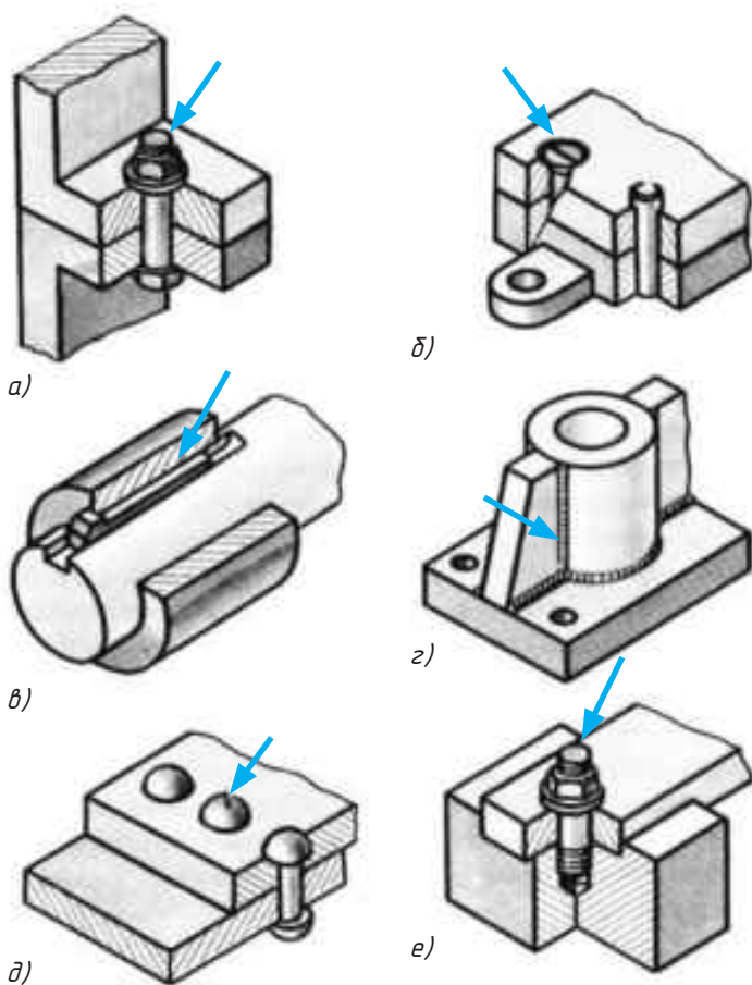
Расми 212. Пайвастҳои гуногуни чузъҳо.
