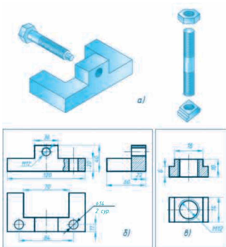
Расми 237. Тасвири аёни ва нақшаҳои ҷузъҳои таъя.
