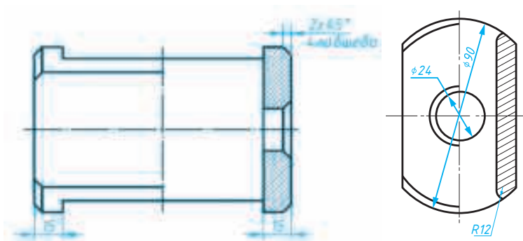
Расми 210. Муфта (бандак).
