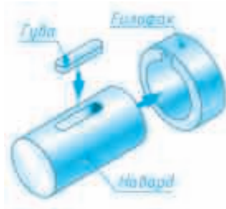
Расми 222. Тасвирҳои аёнии чузъҳои пайвасти гувагӣ.
