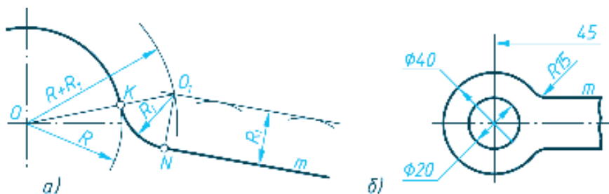
Расми 136. Пайваستاني камони давра бо хати рост.
