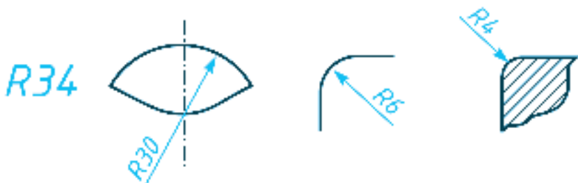
Расми 32. Нишон додани андозаи нимкутр.
