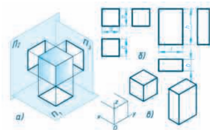
Расми 77: а – проексиясозӣ, б - нақшаҳои мукааб ва параллелепипед, в - проексияи изометрии мукааб.
