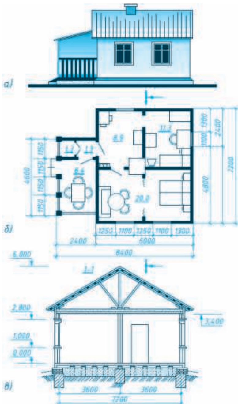
Рисунки 243. Проекты намунави бина.
