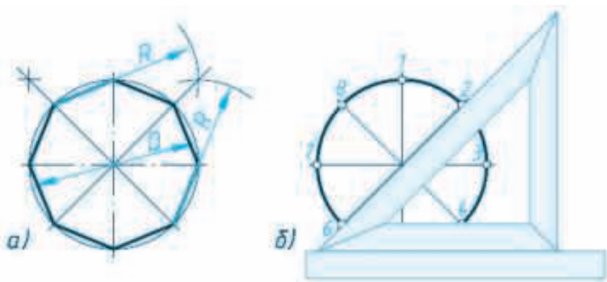
Расми 129. Тақсими давра ба ҳаит ҳиссаи баробар.
