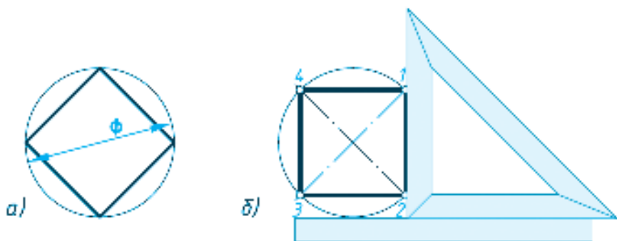
Расми 128. Тақсими давра ба чор ҳиссаи баробар.
