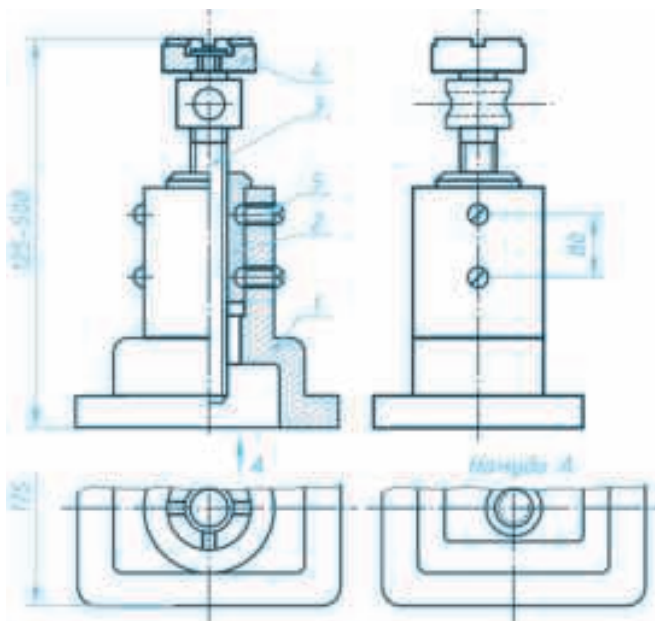
Расми 233. Нақшаи васлияи домкрат.
