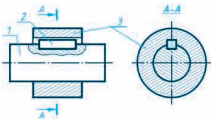
Рисми 224. Нақшаи васлияи пайвасти гувагӣ.
