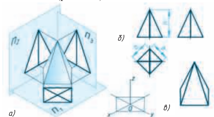
Расми 81: а – проексиясозӣ, б – нақшаи пирамидаи чоркунҷаи мунтазам дар системаи проексияҳои росткунҷа.
