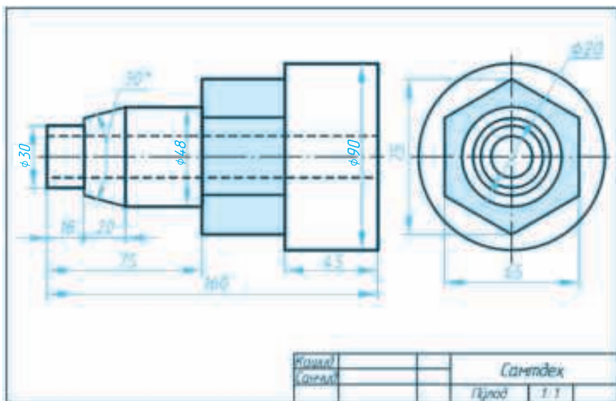
Расми 144. Нақшаи самтдеҳ.
